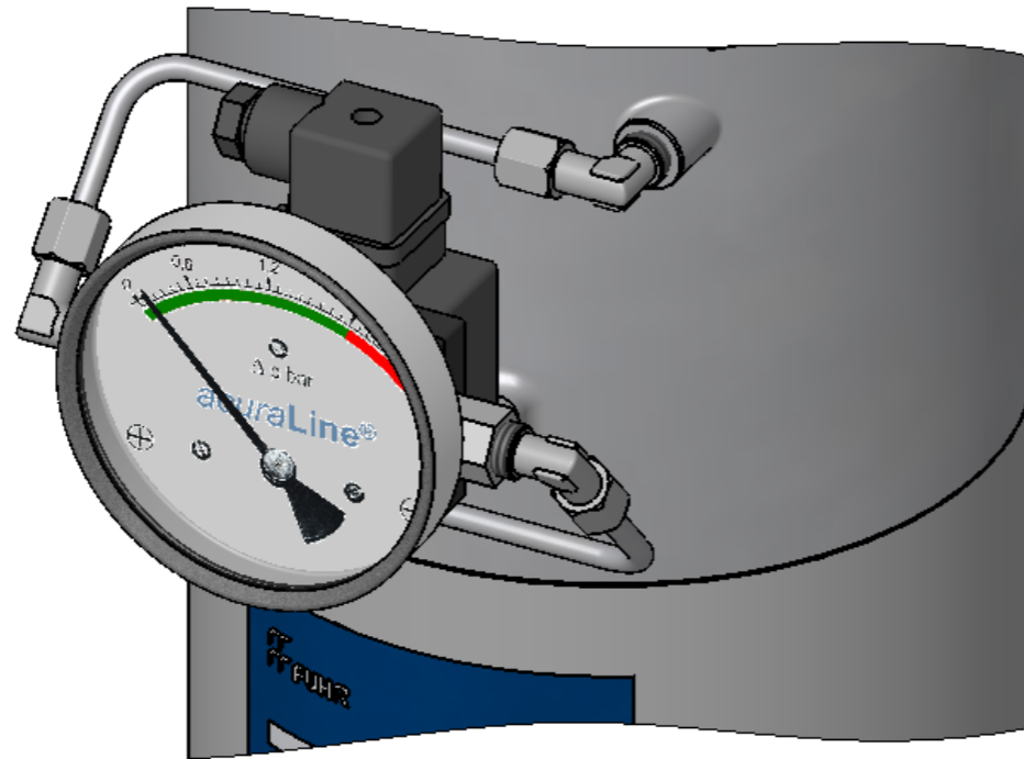
Differenzdruckanzeiger DFA (Abb. mit MG1) nicht im Lieferumfang beinhaltet Differential Pressure Gauge (Illustr. with MG1) not included in differential pressure kit
