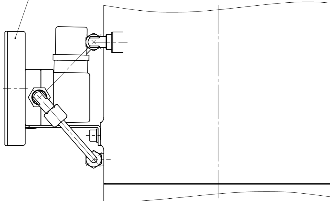
Differenzdruckanzeiger DFA (Abb. mit MG1) nicht im Lieferumfang beinhaltet Differential Pressure Gauge (Illustr. with MG1) not included in differential pressure kit
